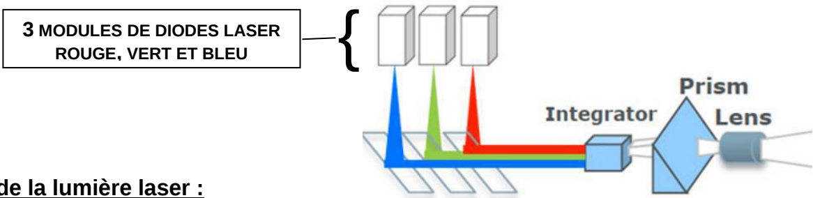
Figure 2 : Schéma de principe de production de lumière blanche du projecteur LASER
