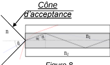
Figure 8 Guidage du laser dans une fibre optique
