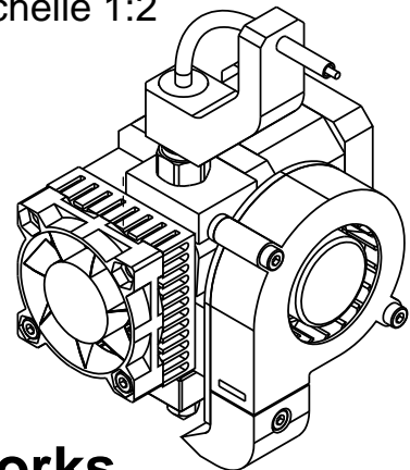
Ensemble monté : Échelle 1:2
